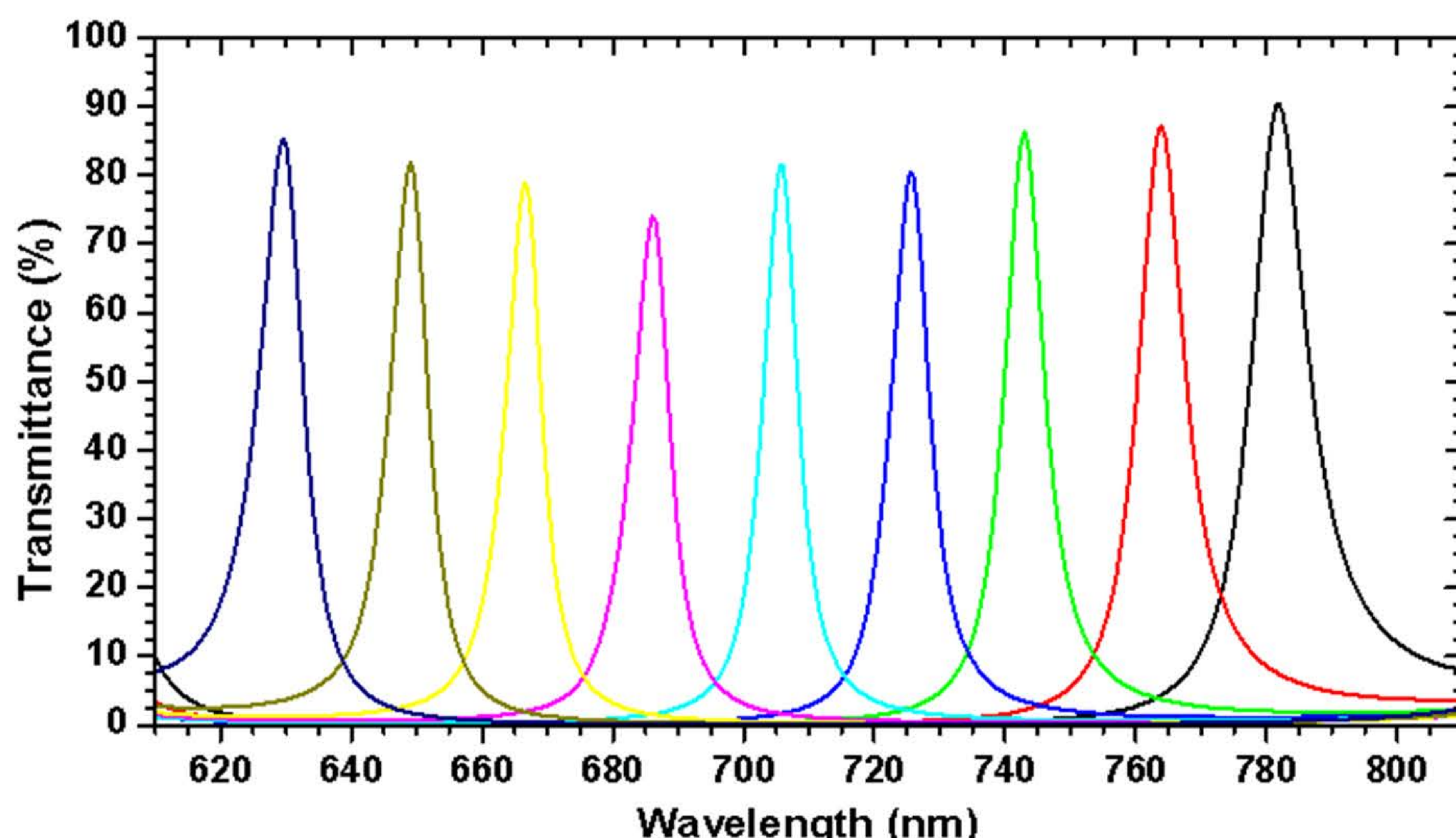
9通道620-800nm波段光谱曲线
